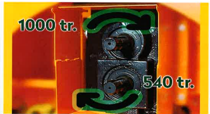
Boîtier inverseur HD intégré 1000/540 tr. Idéal pour le montage en position frontale
